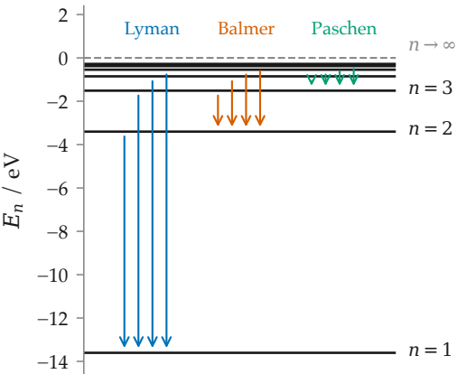
Niveles del átomo de hidrógeno
