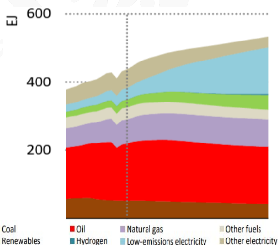
Gráfica 1. Consumo final por combustible en escenario de políticas actuales, 2010 - 2050
