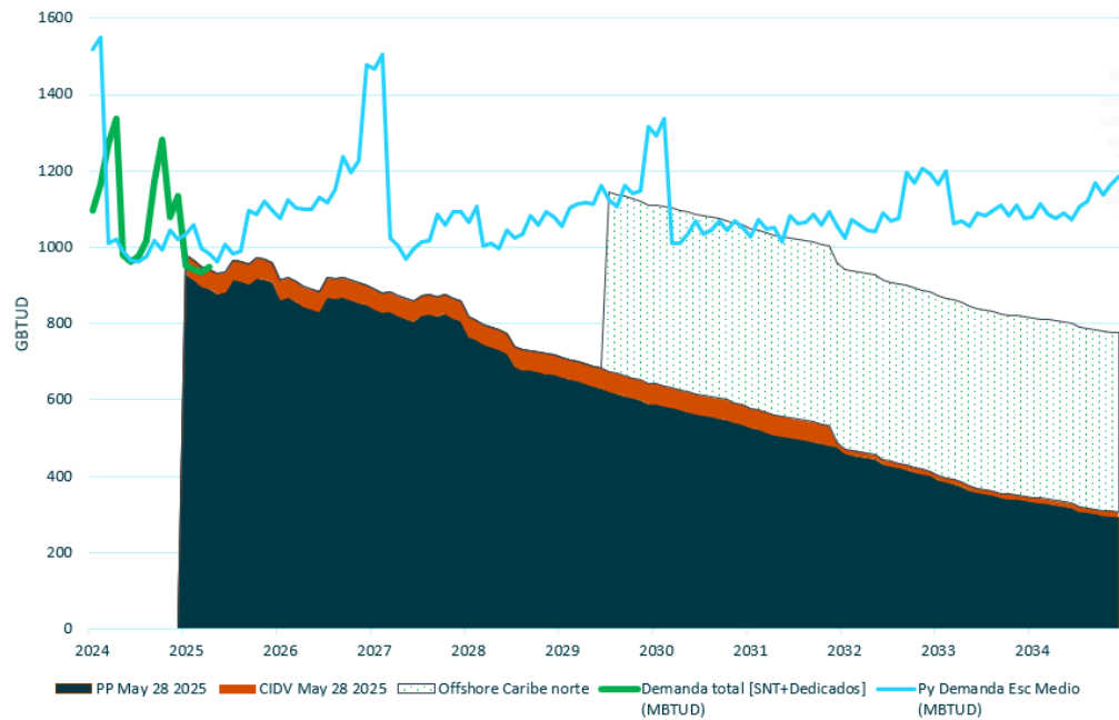
Gráfica 19. Balance volumétrico de gas natural 2025 – 2034 + offshore
