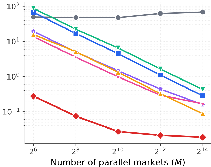
Time per agent-event (ns, log scale)
