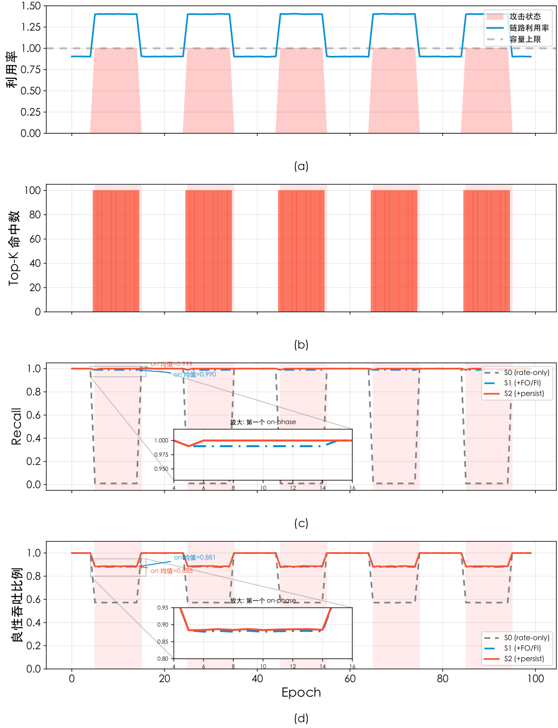
图 3-4 脉冲式 on-off 攻击下的时域响应 ( M = 100 )。 (a) 目标链路利用率; (b) 一级候选命中中的攻击 key 数量; (c) 不同方案的 Recall; (d) 不同方案的良性吞吐比例
