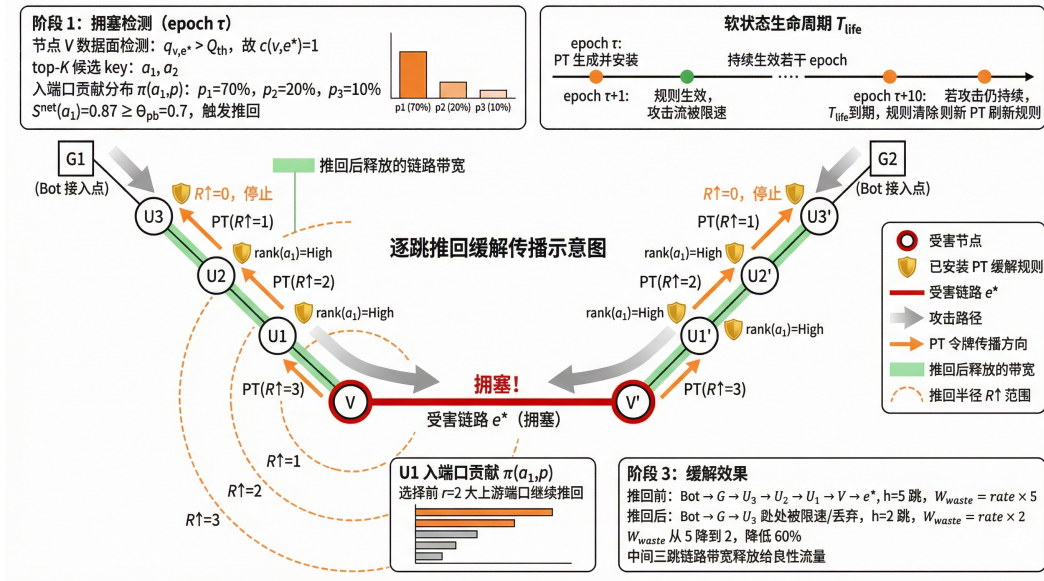
图 4-3 逐跳推回过程示意。(a) 拥塞检测与入端口贡献分布; (b) PT 令牌逐跳推回; (c) 软状态生命周期; (d) 推回前后的 W_{waste} 对比
