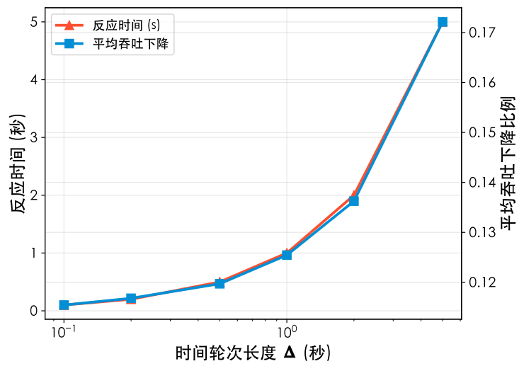
图 3-7 epoch 长度 \Delta 对反应时间与良性吞吐下降的影响 ( M = 100 , S1 方案)
