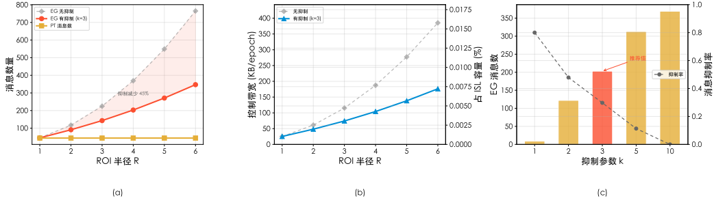
图 4-6 协同控制开销与抑制机制效果。(a)EG 消息数随 R 变化；(b) 控制带宽随 R 变化；(c) 抑制参数 k 的影响
