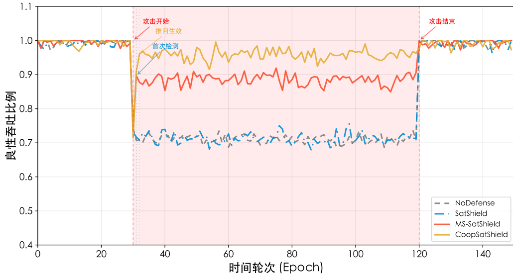
图 4-5 良性吞吐随时间变化 ( M = 100 )
