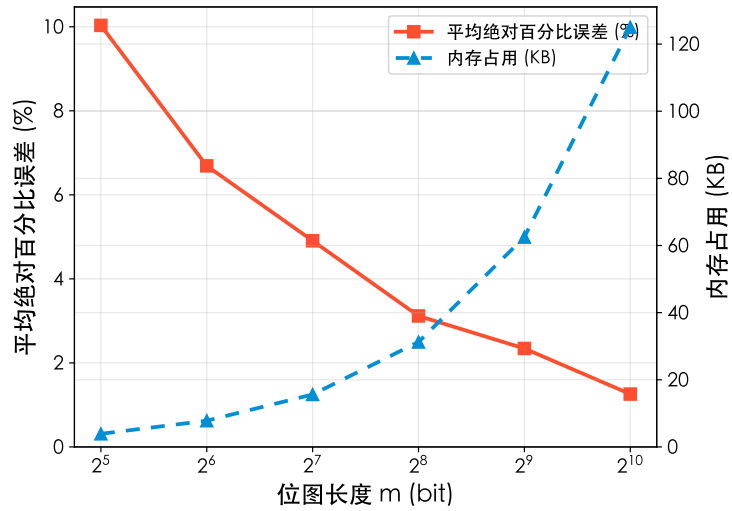
图 3-6 位图长度 m 对 FI/FO 估计误差与总内存的影响（ M = 100 ，S1 方案）
