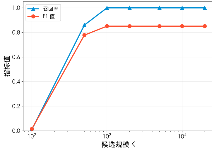
图 3-5 候选规模 K 对 Recall 与 F1 的影响（ M = 100 ，S1 方案）
