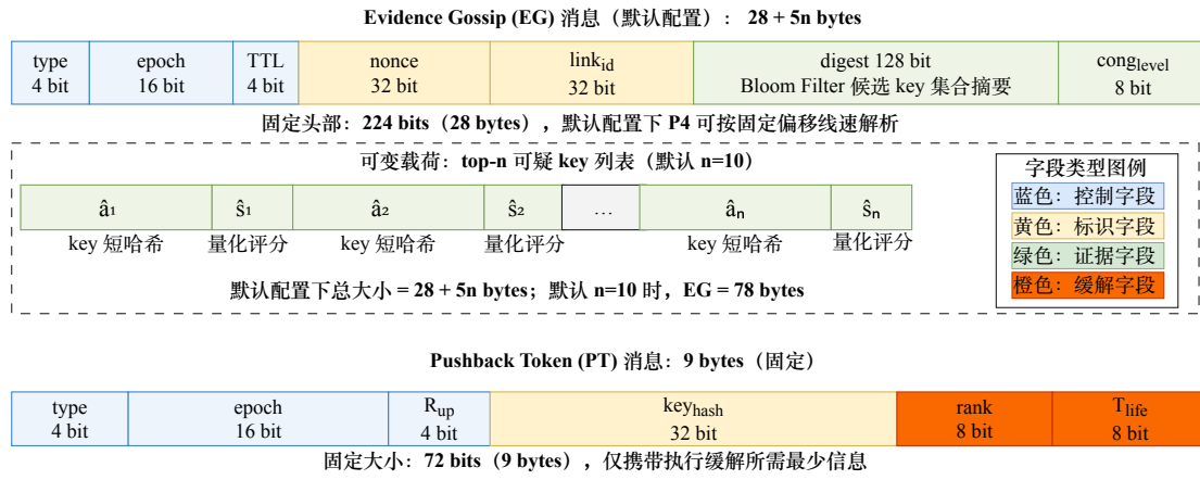
图 4-2 EG/PT 协同控制消息格式 (默认配置)。上: Evidence Gossip (EG) 消息; 下: Pushback Token (PT) 消息
