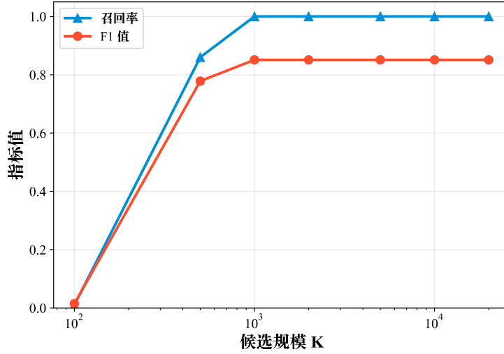
图 3-5 候选规模 K 对 Recall 与最终识别 F1 的影响
