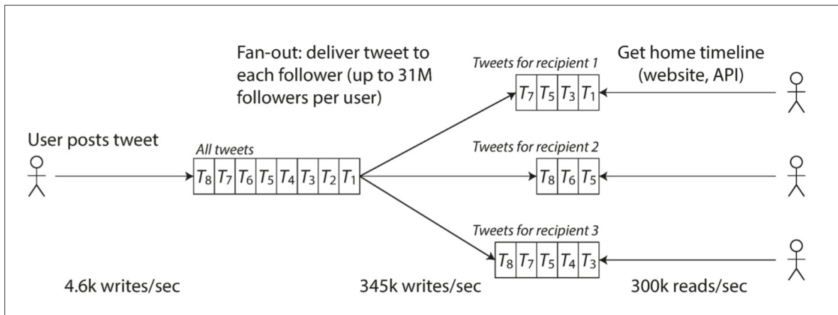
图1-3 用于分发推特至关注者的数据流水线，2012年11月的负载参数【16】
