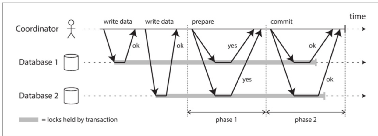
图9-9 两阶段提交（2PC）的成功执行
