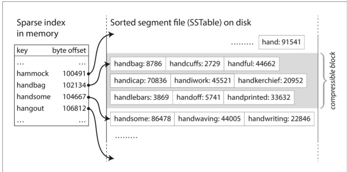
图3-5 具有内存索引的SSTable
