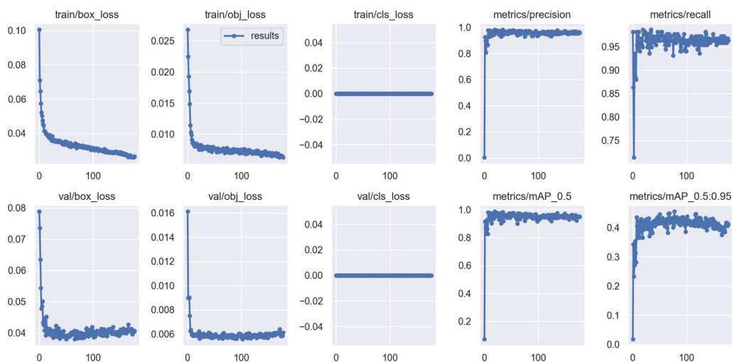
YOLOv5 训练曲线
