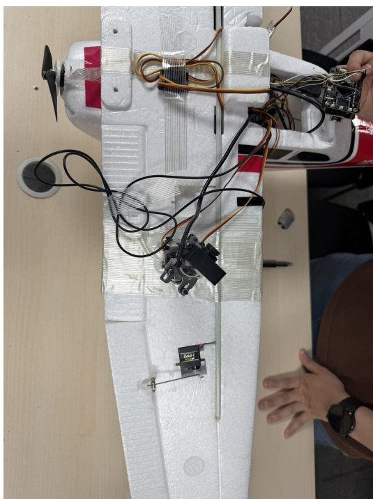
图 4.1 已组装固定翼无人机的任务载荷与舵机
