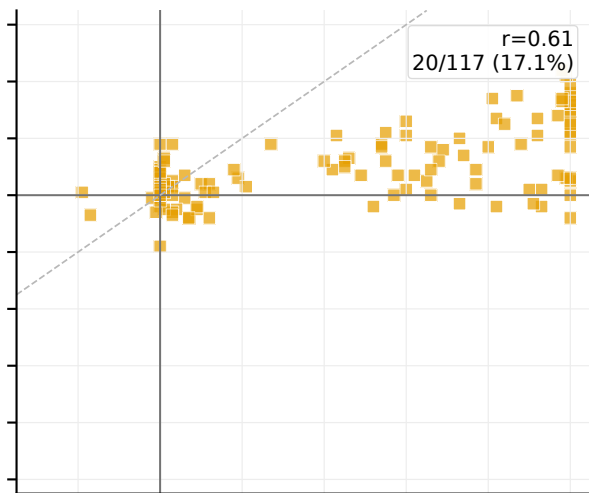
StrategyQA
