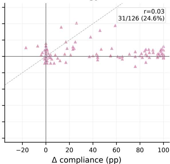
StrategyQA
