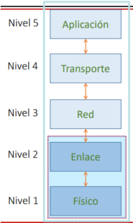
Figura 2.13: Pila de protocolos TCP/IP
