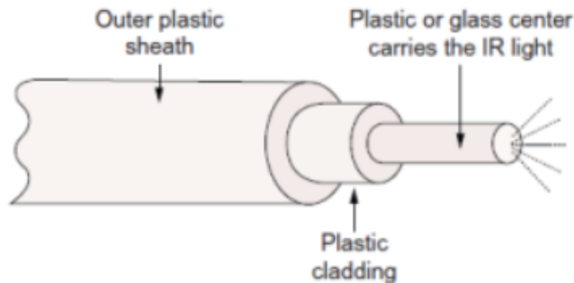
Figura 1.13: Ejemplo de fibra óptica
