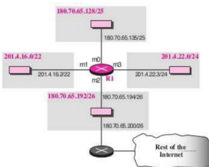
Figura 5.3: Topología de red del ejemplo con routers
