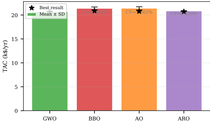
Mean \pm SD TAC over 30 runs Case~4 (PV--BESS--SC--Grid)
