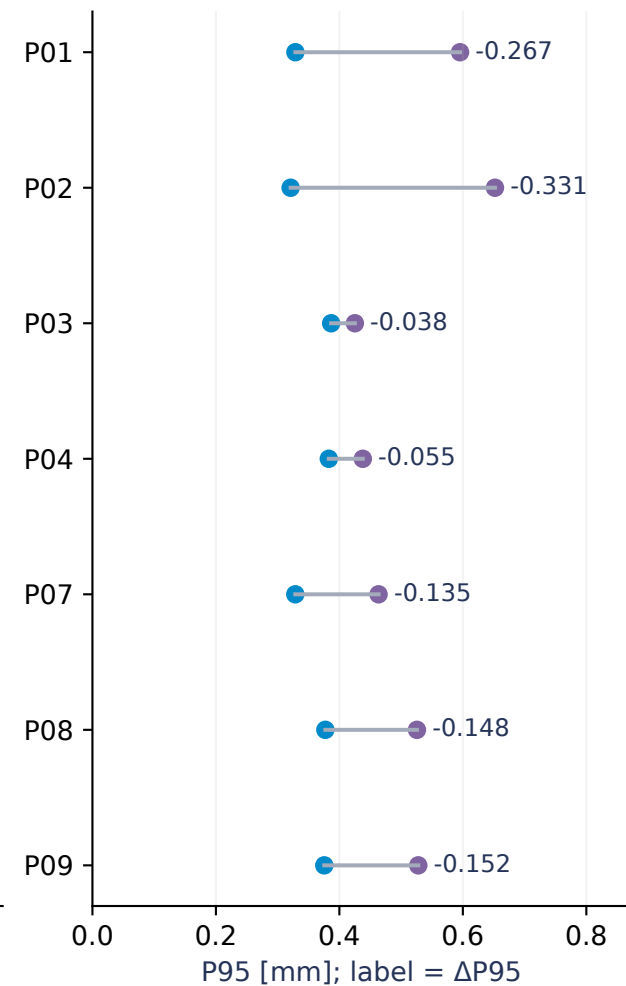
B Paired P95
