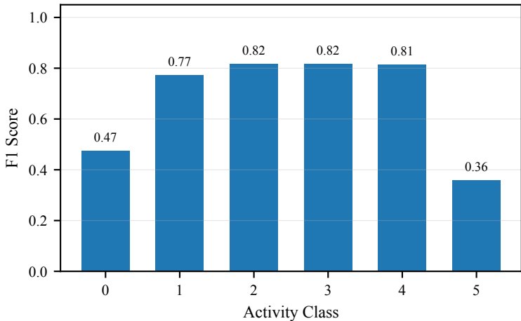
Per-Class Test F1 Score
