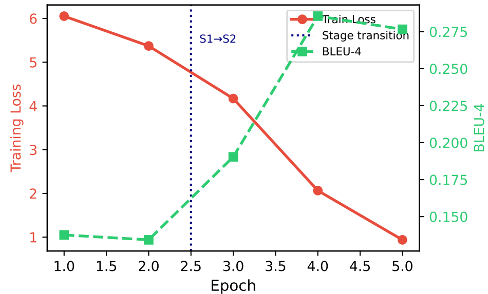
DAMF (Ours)
