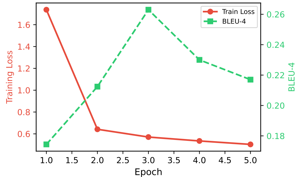
Naïve FT
