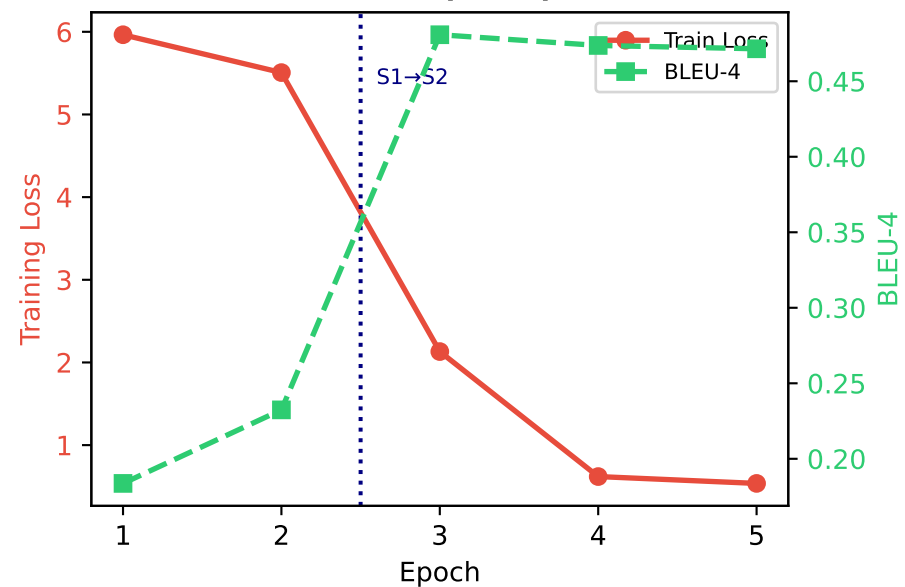
DAMF (Ours)
