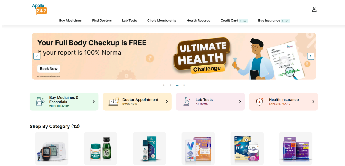
Fig 4: 04_after_login
