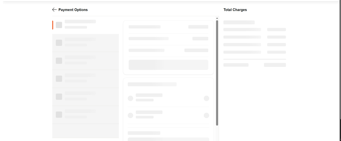
Fig 15: 14_proceed_to_pay
