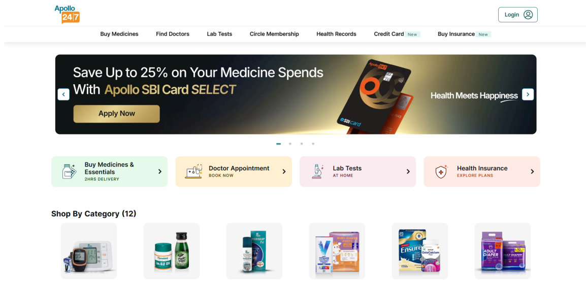
Fig 1: 01_homepage
