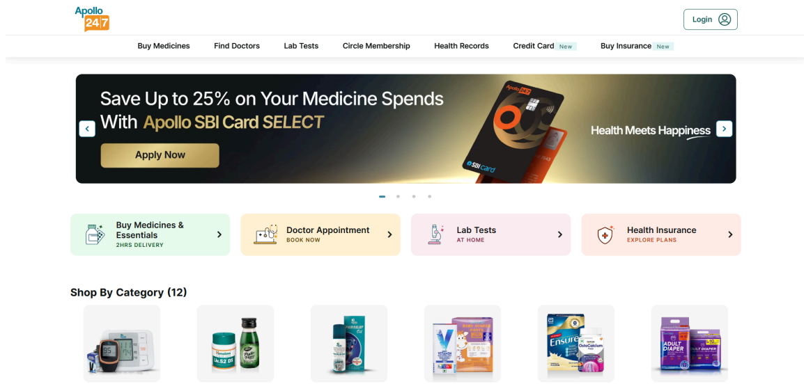
Fig 1: 01_homepage
