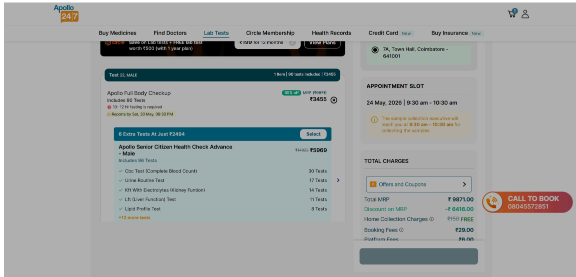
Fig 15: 14_proceed_to_pay
