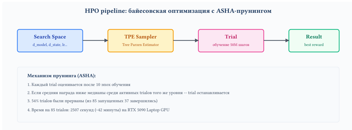
Рисунок 10 — НРО pipeline
