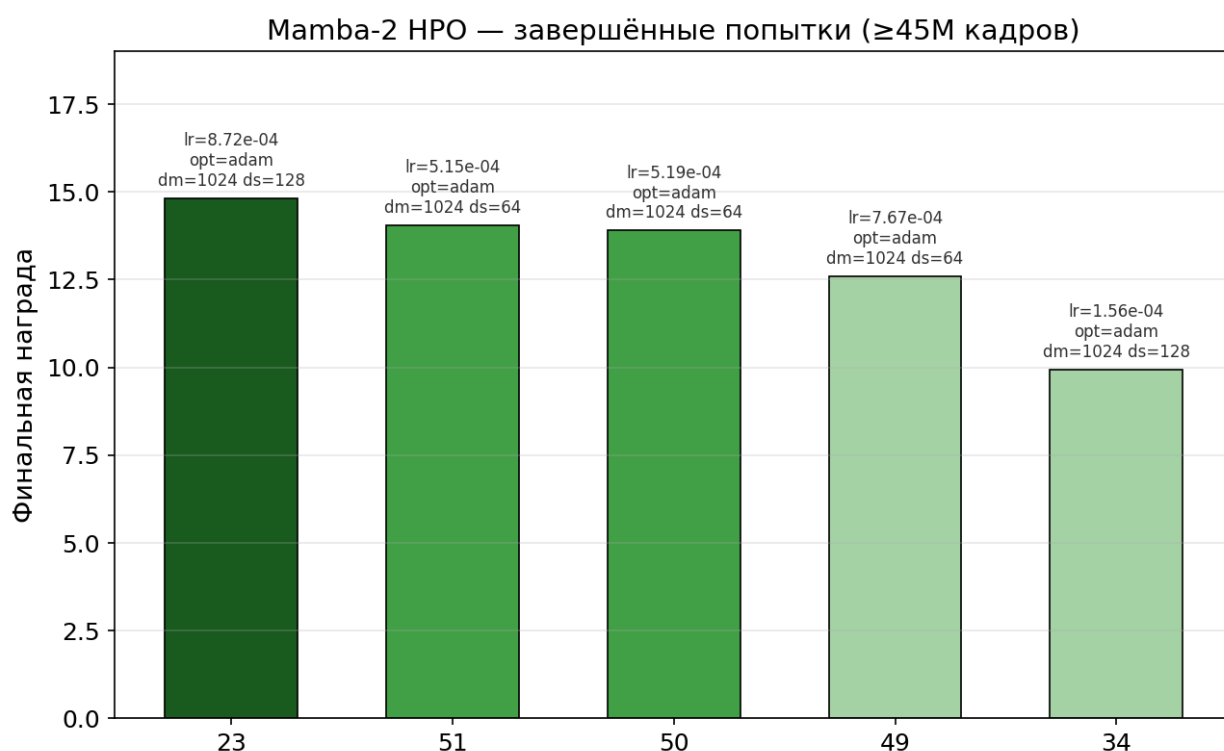
Рисунок 11 — Топ-5 завершённых trials НРО для Mamba-2 с конфигурациями
