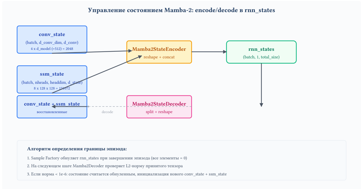
Рисунок 7 — Кодирование и декодирование состояния Mamba-2
