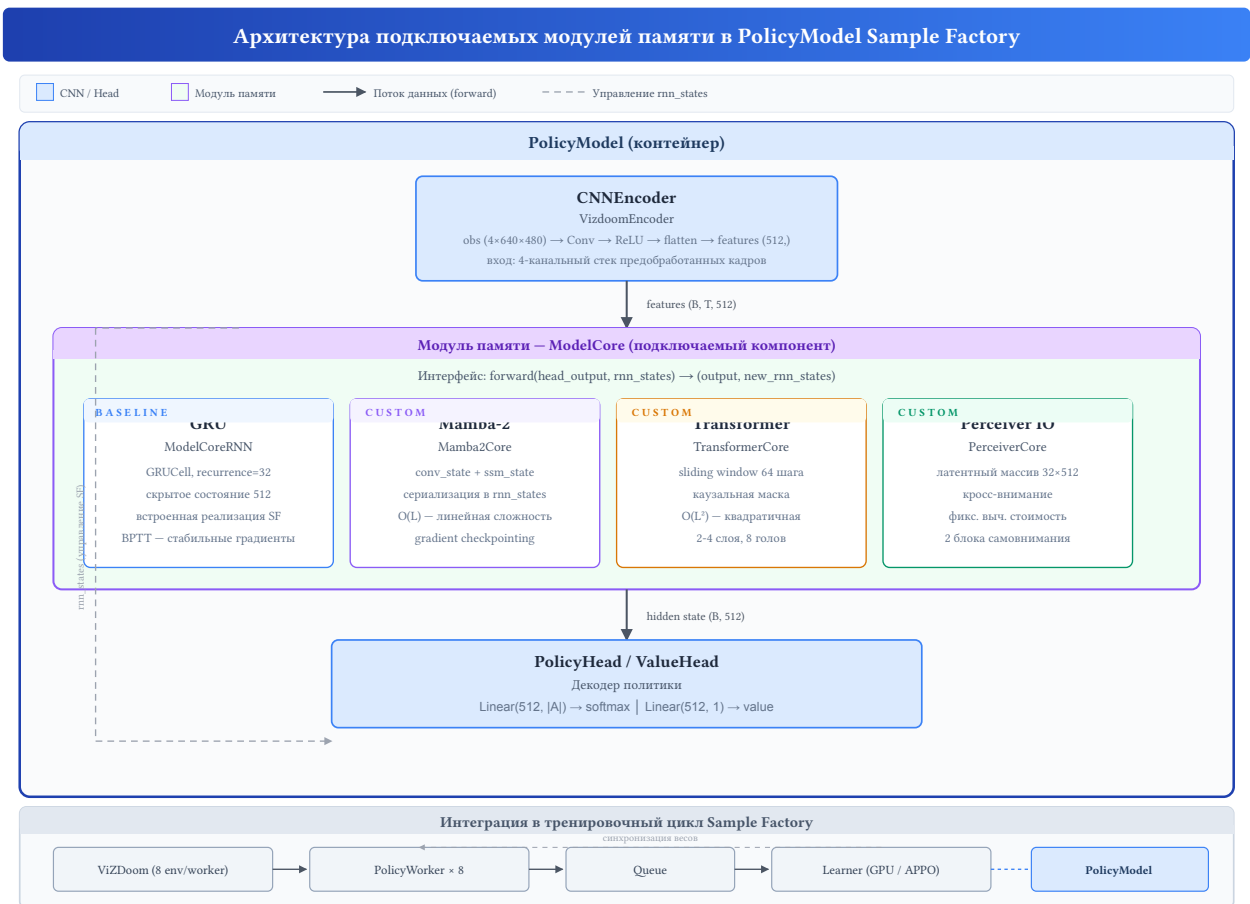
Рисунок 6 — Архитектура PolicyModel со сменным модулем памяти
