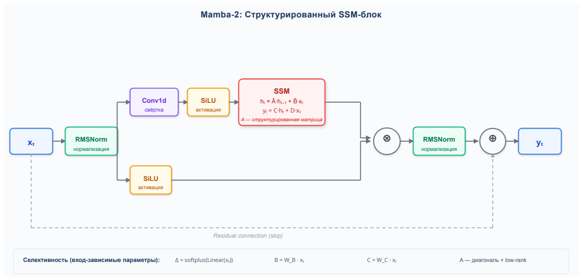
Рисунок 4 — Структура SSM-блока Mamba-2
