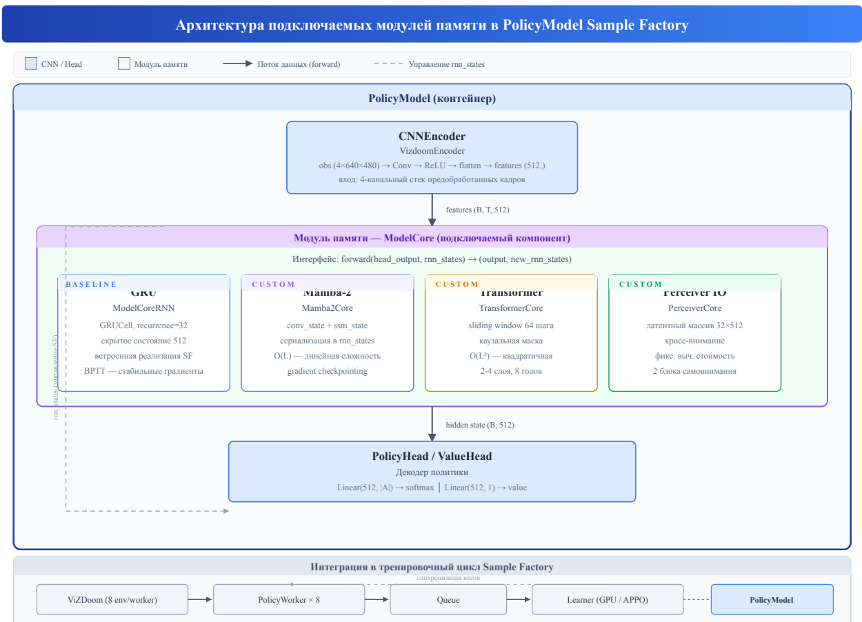
Рисунок 6 — Архитектура PolicyModel со сменным модулем памяти: GRU, Mamba-2, Transformer и Perceiver IO. CNNEncoder и PolicyHead/ValueHead фиксированы. Интеграция в тренировочный цикл Sample Factory.
