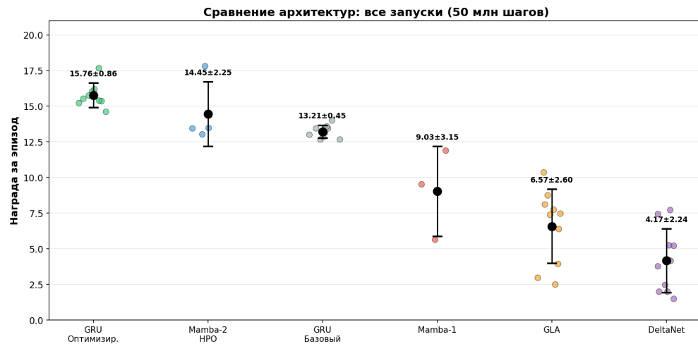
Рисунок 24 — Scatter-график всех архитектур: каждый seed — точка
