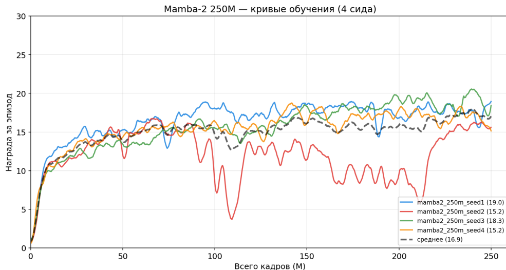
Рисунок 21 — Mamba-2 250M: 4 сида
