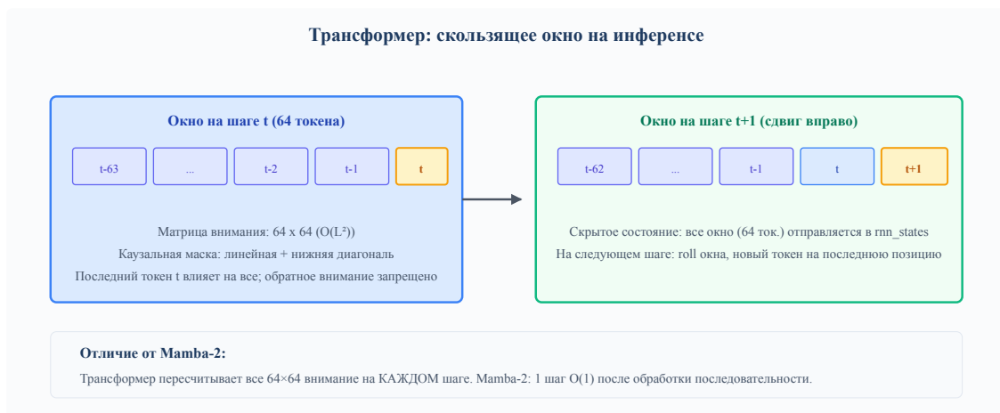
Рисунок 9 — Скользящее окно TransformerCore на инференсе
