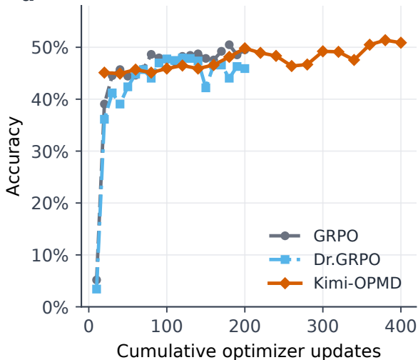
a Accuracy per optimizer update
