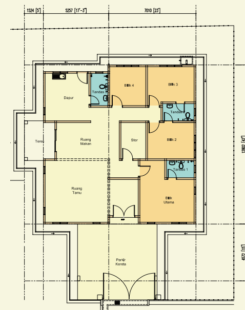
Pelan Lantai
