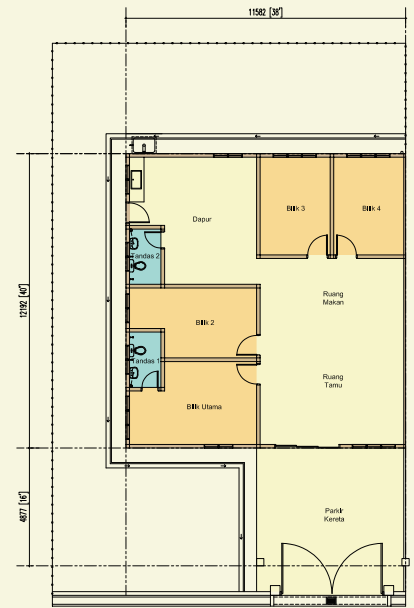
Pelan Lantai
