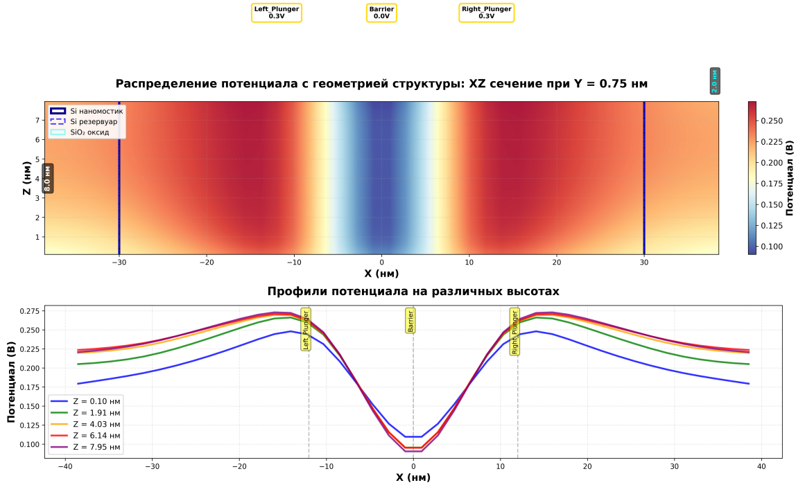
Рис. 4.2. Распределение электростатического потенциала в поперечном сечении наномостика для конфигурации двойной квантовой точки (Double Quantum Dot) по архитектуре Loss-DiVincenzo. Структура содержит три затворных электрода: левый и правый плунжерные затворы (Left/Right Plunger) с потенциалом 0.3 В и центральный барьерный затвор (Barrier) с потенциалом 0 В.
