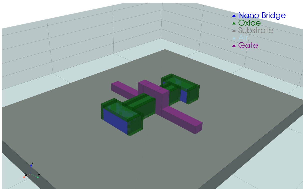
Рис. 3.1. Структура на которой показаны возможности программного задания модели. Есть возможность задавать нанопровод с утолщениями по краям (синий цвет), оксид на этом нанопроводе (зеленый цвет), а также затворный элетрод с оксидом на нем (фиолетовый цвет)
