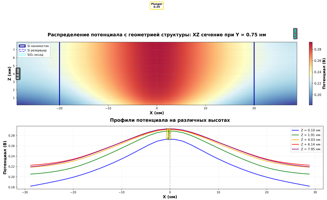
Рис. 4.1. Распределение электростатического потенциала в поперечном сечении наномостика для конфигурации одиночной квантовой точки. Структура содержит один затворный электрод с потенциалом 0.3 В, расположенный в центре наномостика.
