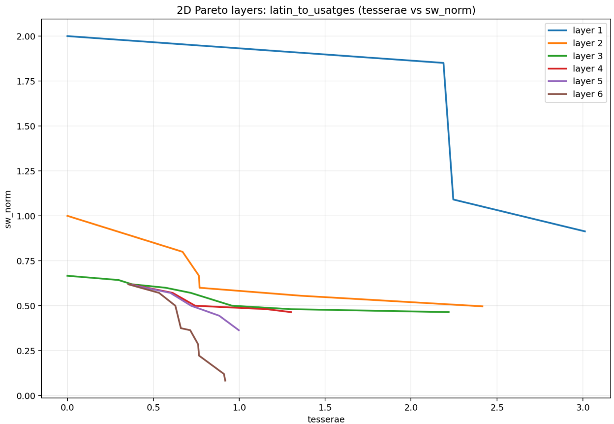
Рисунок 1.2 — Двумерные парето-слои для эксперимента «латинские источники → Барселонские обычаи» в пространстве мер Tesseractae и SW_{\text{norm}}
