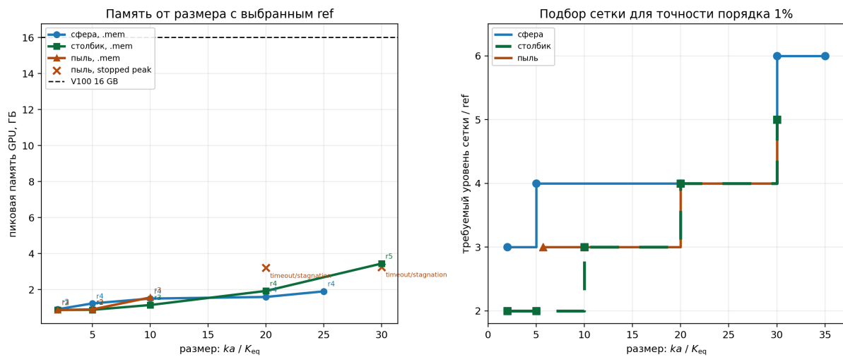
Рис. 21.1: Экспериментальная зависимость видеопамяти от размера и дискретизации. Линии следует интерпретировать только в пределах измеренного диапазона; форма и качество сетки изменяют число RWG при одинаковом ka .
