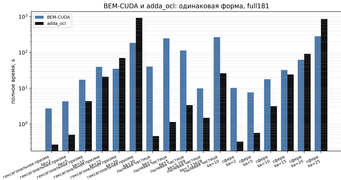
Рис. Ф.9: Сравнение вычислительных backend-ов при согласованной физической задаче.
