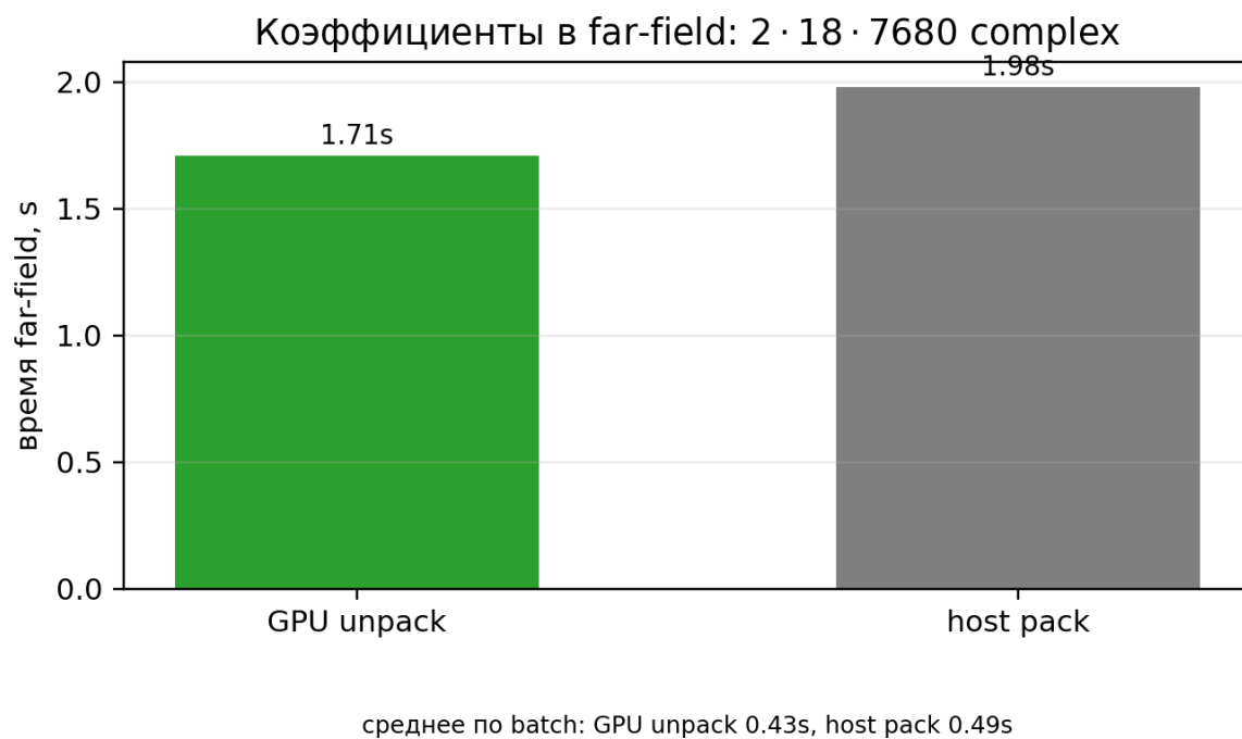
Рис. F.13: Накладные расходы передачи коэффициентов токов на GPU.
