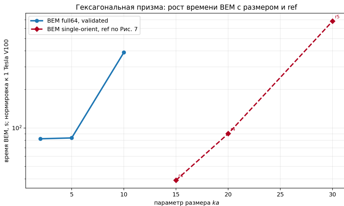
Рис. Ф.7: Измеренное время расчёта призмы.
