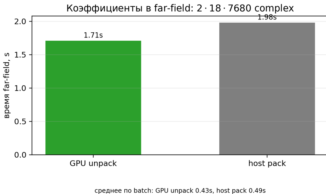
Рис. Г.13: Накладные расходы передачи коэффициентов токов на GPU.
