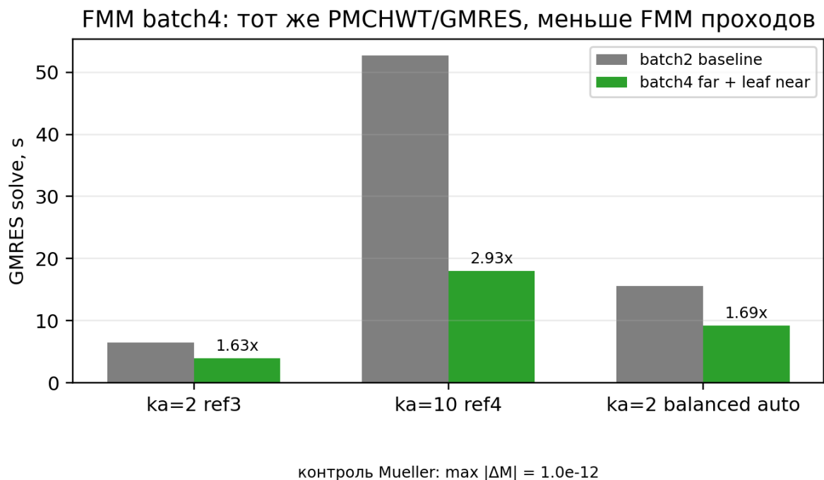
Рис. 23.2: Эффект пакетного вычисления двух токов и двух поляризаций. Ускорение относится к конкретной версии ядра и не заменяет контроль итоговой невязки.
