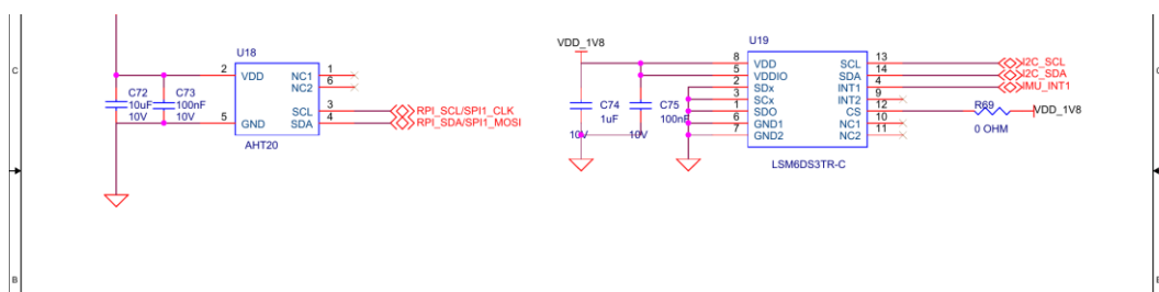
图 2-7 AHT20 与 IMU 相关原理图
