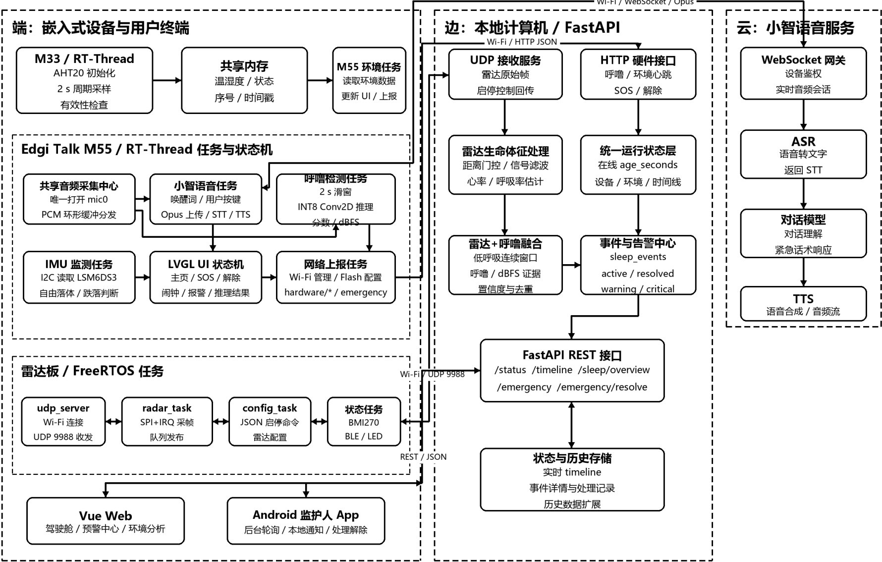
多模态睡眠看护系统端—边—云软件架构
