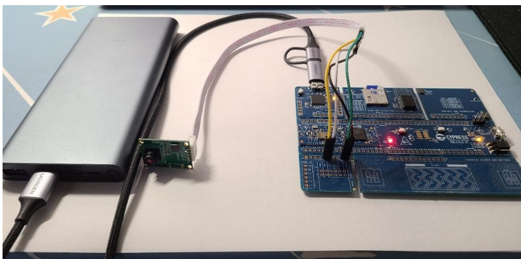
图 3-2 系统实物全局连接示意（二）
