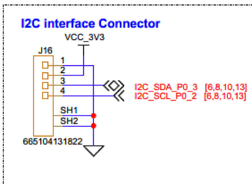
图 2-8 I2C 接口连接器原理图
