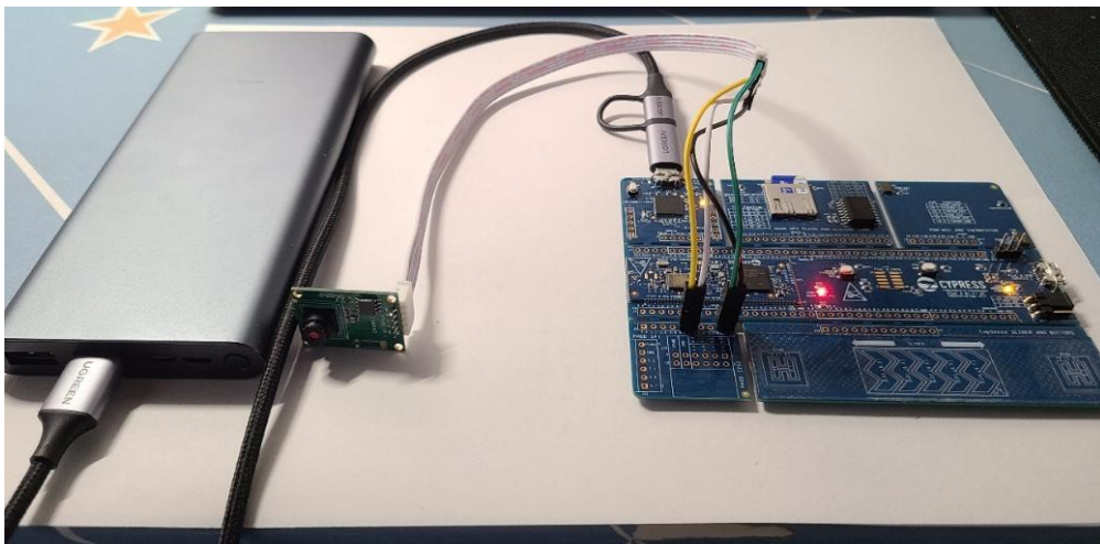
图 2-3 雷达模块测试摆放场景
