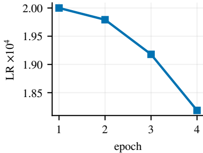
Cosine LR
