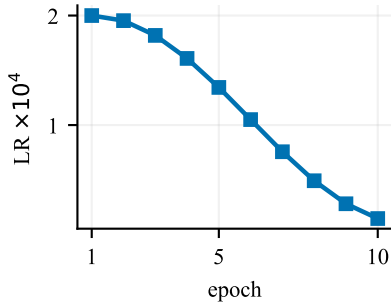
Cosine LR
