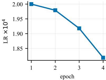
Cosine LR
