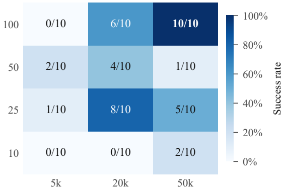
Diffusion Policy (v2)
