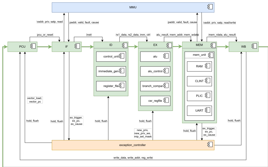
Рис. 2: Структурная схема соединения Verilog-модулей процессорного ядра
