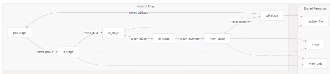
Рис. 2: Структурная схема соединения Verilog-модулей процессорного ядра
