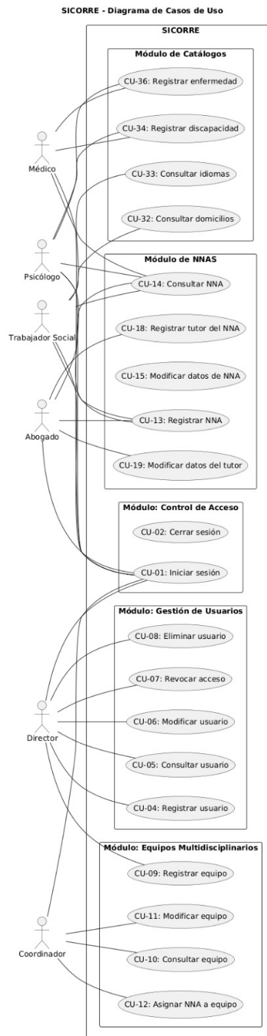
Figura 3.1: Diagrama de subsistemas y casos de uso.
