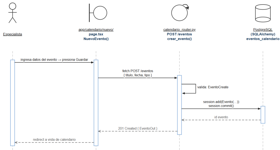
Figura 4.39: Diagrama de secuencia — CU-39 Registrar evento en calendario.
