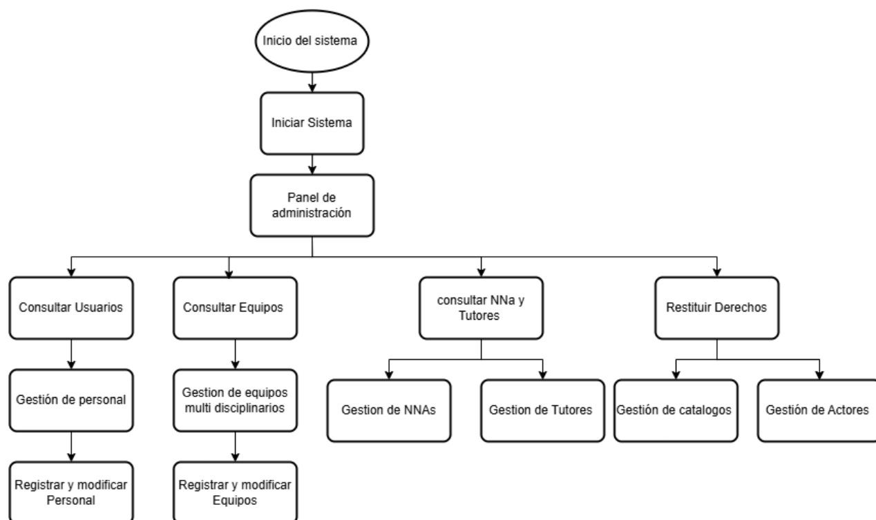
Figura 5.1: Mapa de navegación del sistema SICORRE.
