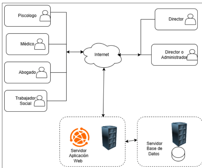
Figura 2.3: Arquitectura del sistema.
