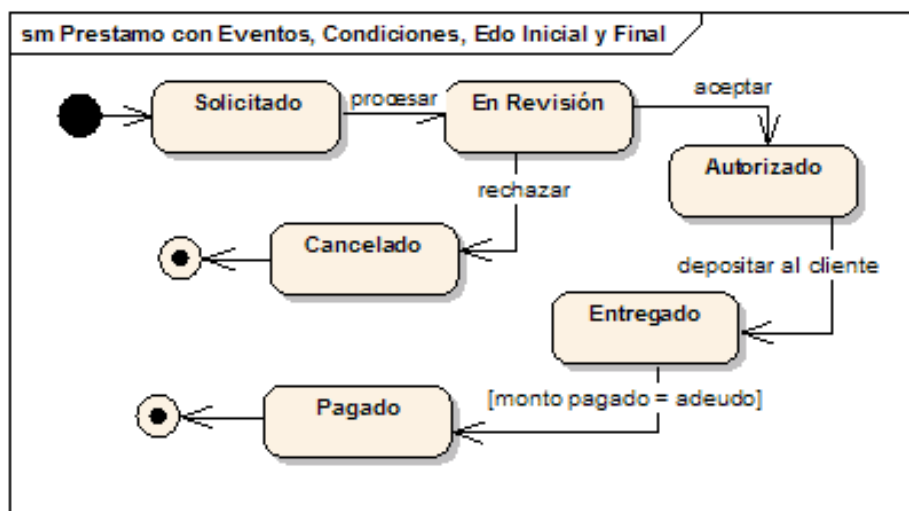
Figura 3.2: Máquina de estados de un Préstamo.
