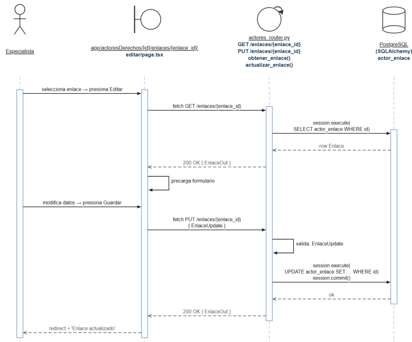
Figura 4.53: Diagrama de secuencia — CU-53 Editar enlaces representantes.
