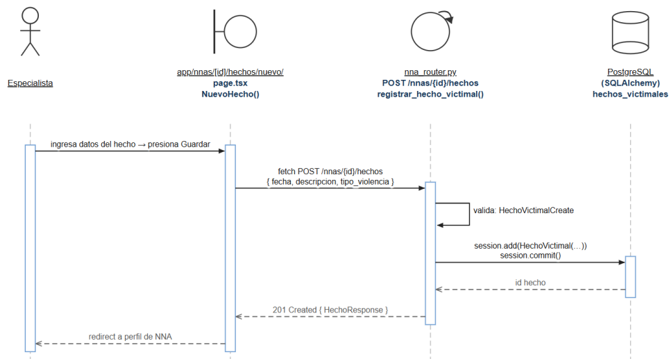
Figura 4.16: Diagrama de secuencia — CU-16 Registrar hecho victimal.
