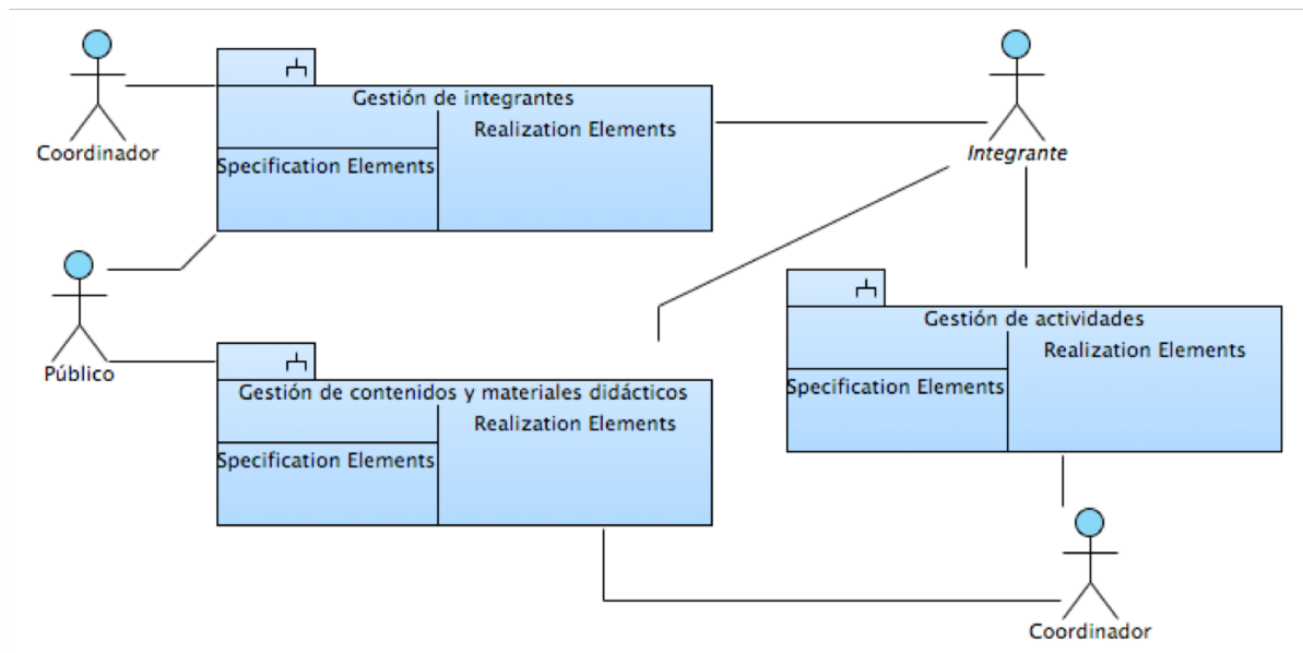
Figura 3.1: Diagrama de subsistemas y casos de uso.
