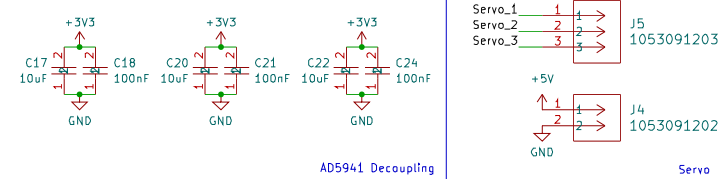
AD5941 Decoupling
