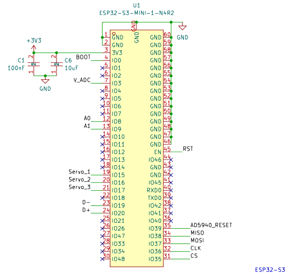
ESP32-S3
