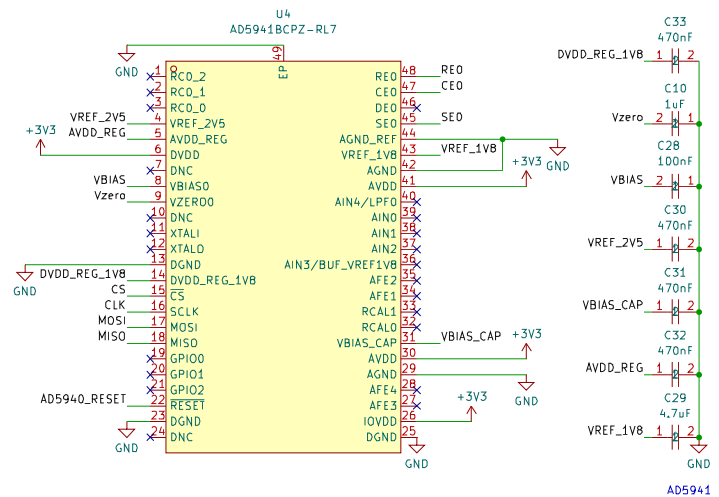
AD5941
