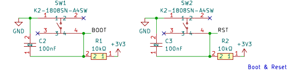
Boot & Reset
