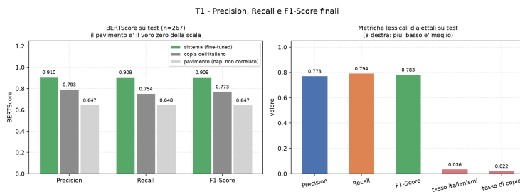
Figura 3: Grafico di confronto metriche Precision, Recall e F1-Score per il Fine-Tuning sulla Traduzione in dialetto Napoletano
