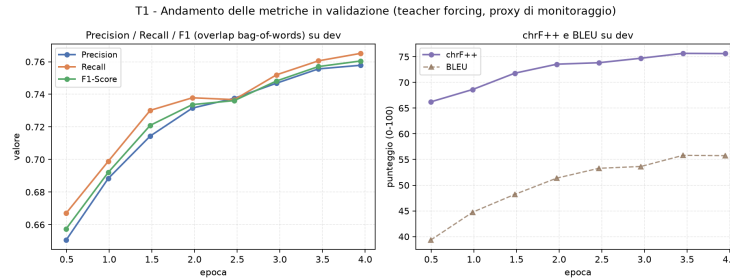
Figura 2: Grafico andamento delle metriche Precision, Recall e F1-Score per il Fine-Tuning sulla Traduzione in dialetto Napoletano
