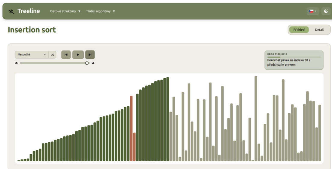
Obrázek 7.2: Obecný přehled třídícího algoritmu s využitím sloupkové vizualizace
