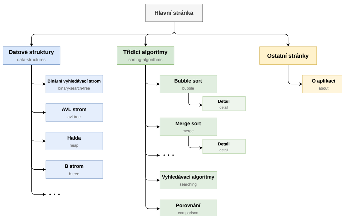
Obrázek 6.1: Sitemap aplikace, znázorňující hierarchii stránek a jejich vzájemné propojení
