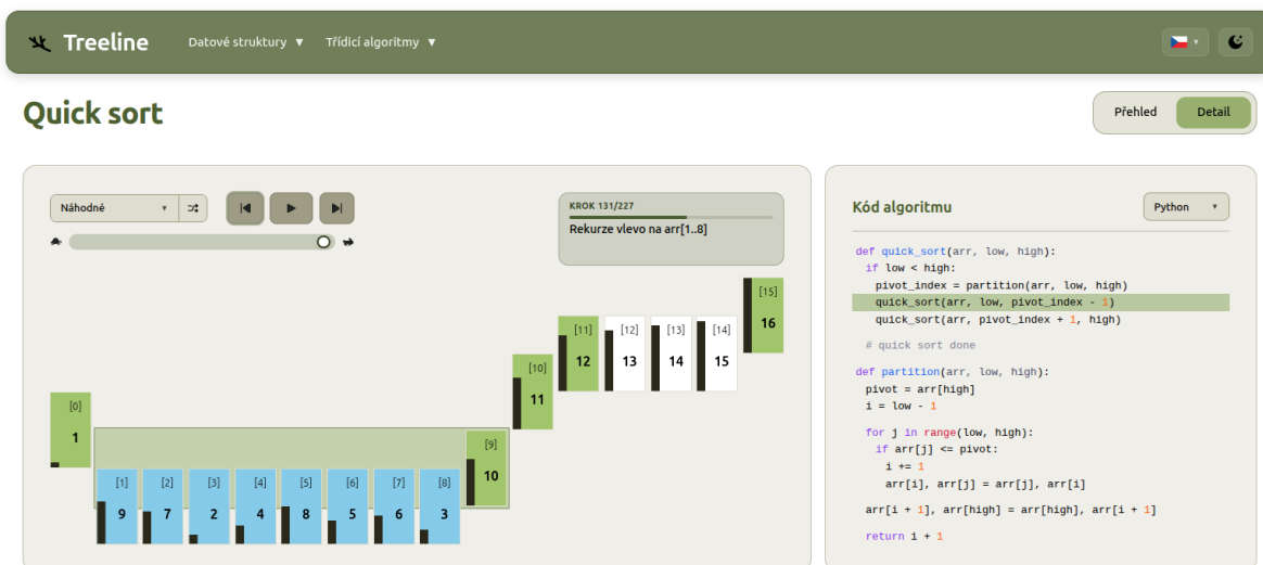
Obrázek 7.3: Detailní pohled rekursivního algoritmu Quick Sort
