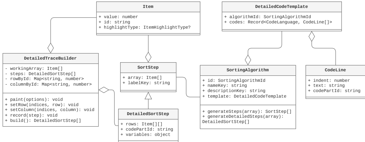
Obrázek 6.10: Diagram tříd pro reprezentaci třídících algoritmů
