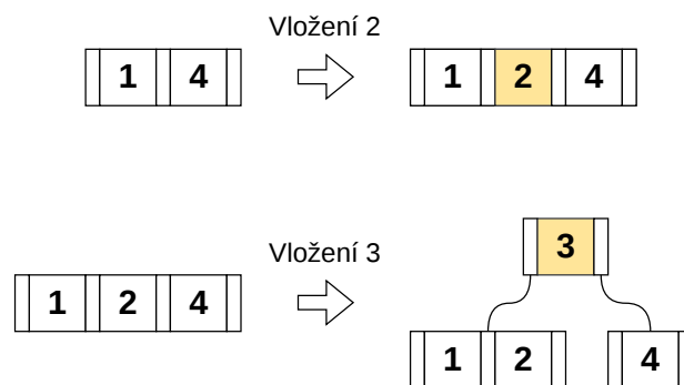
Obrázek 2.10: Vložení klíče do B-stromu řádu 4
