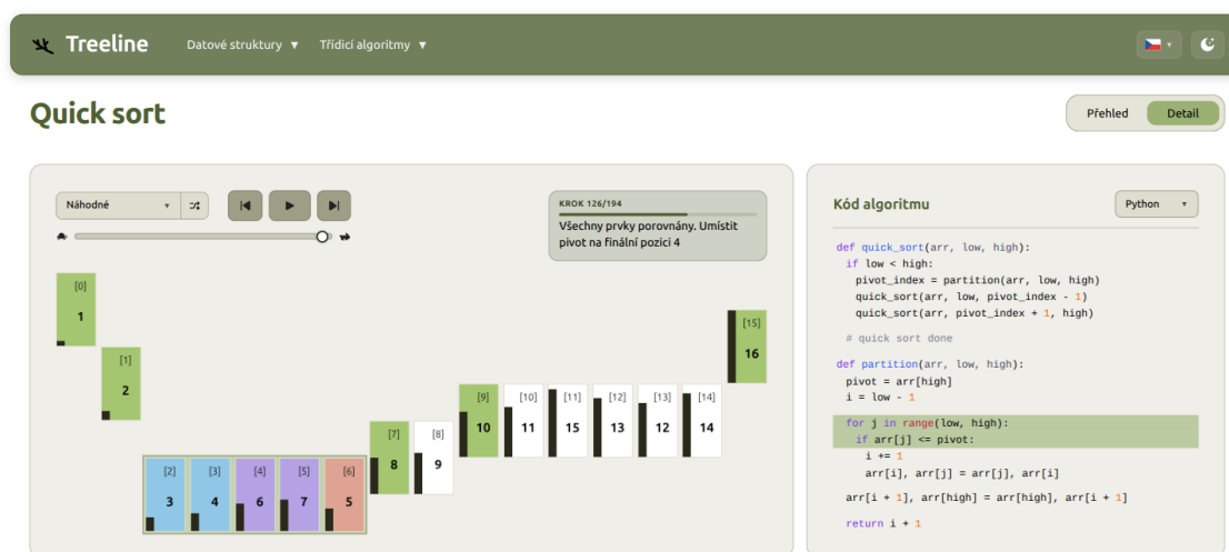
Obrázek 7.3: Detailní pohled rekurzivního algoritmu s dynamickým mapováním pseudokódu
