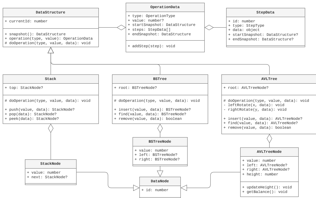
Obrázek 6.9: Diagram tříd pro reprezentaci datových struktur
