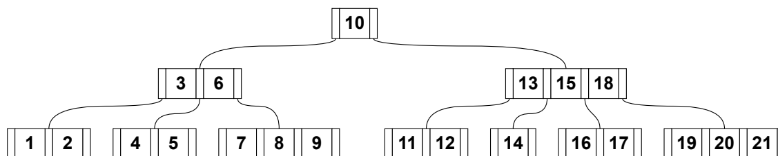
Obrázek 2.9: B-strom řádu 4
