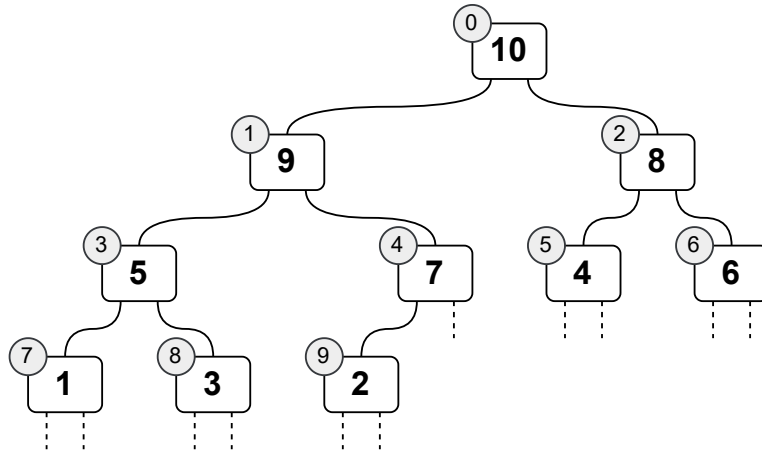
Obrázek 2.11: Binární halda reprezentovaná stromem
