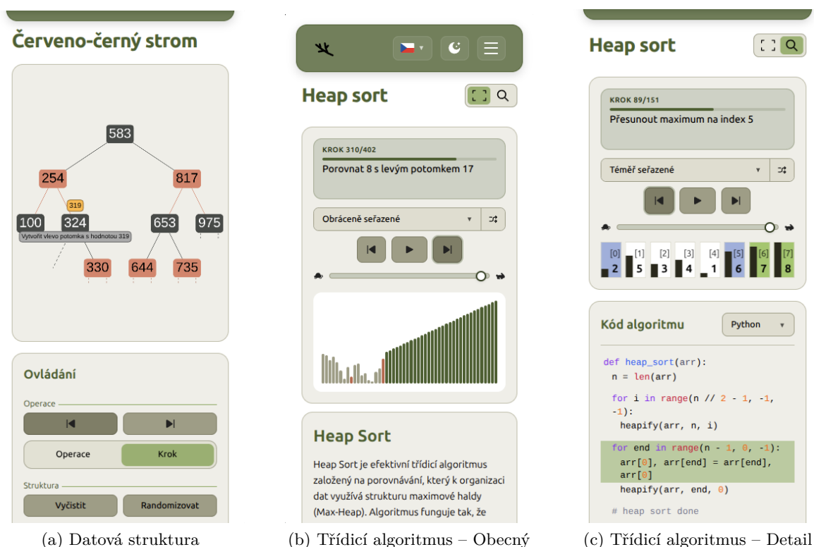
Obrázek 7.4: Ukázka responzivního chování na mobilním zařízení
