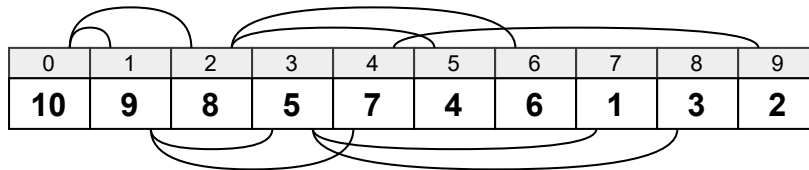
Obrázek 2.12: Binární halda reprezentovaná polem
