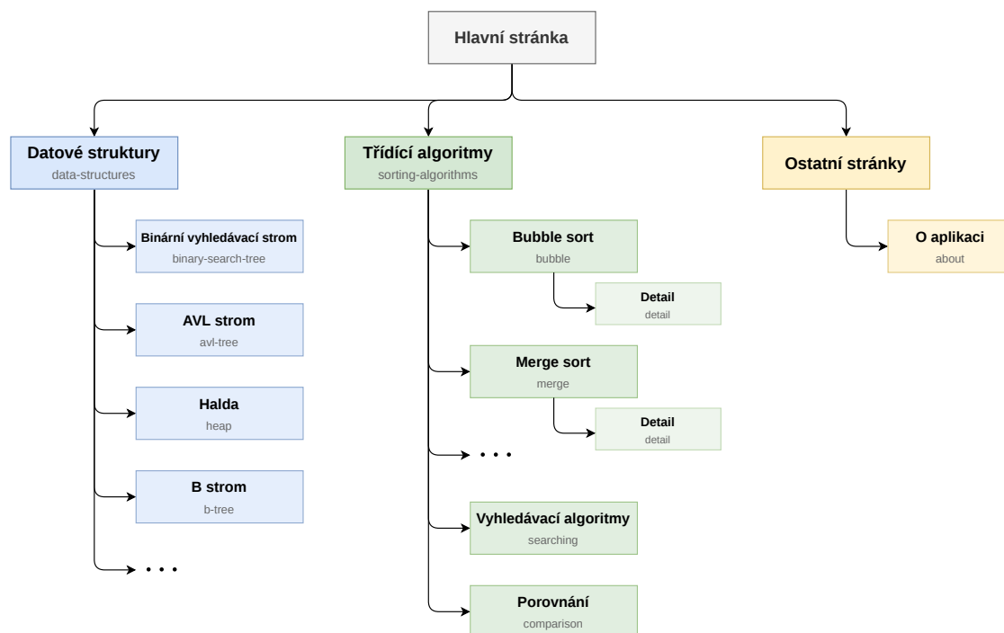
Obrázek 6.1: Sitemap diagram aplikace znázorňující hierarchii stránek a jejich propojení
