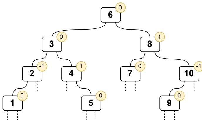
Obrázek 2.4: AVL strom
