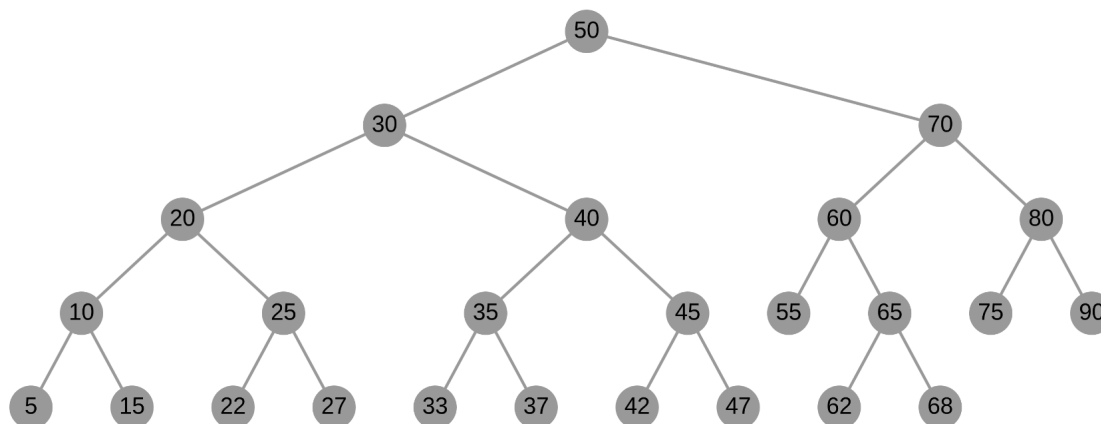
Obrázek 5.4: Příklad vykreslení stromu pomocí knihovny Cytoscape.js
