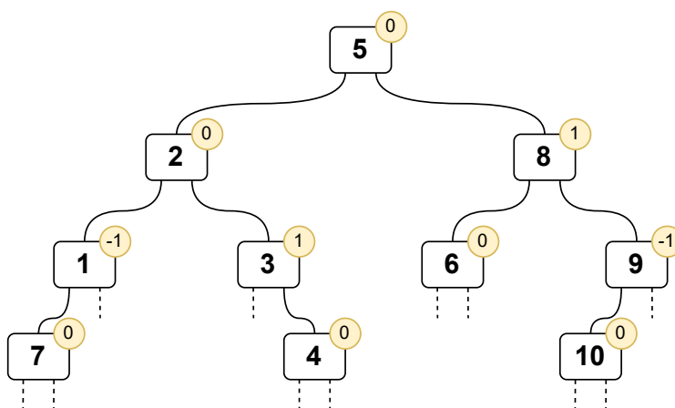
Obrázek 2.4: AVL strom
