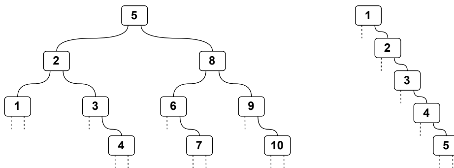
Obrázek 2.3: Binární vyhledávací strom
