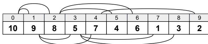
Obrázek 2.12: Binární halda reprezentovaná polem
