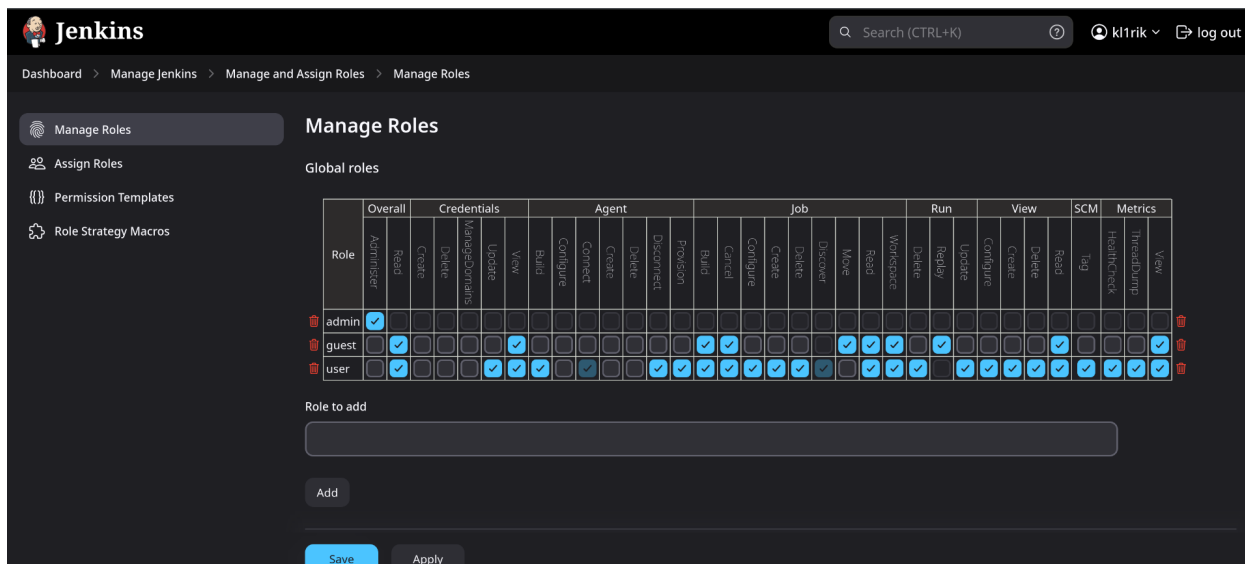
Рисунок 1.2 – Настройка механизма контроля доступа с помощью плагина RBAC
